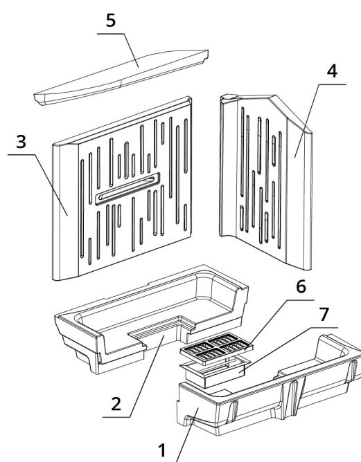
Carcon Feuerraum
